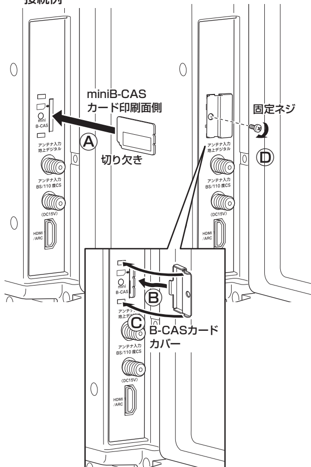
接続例
