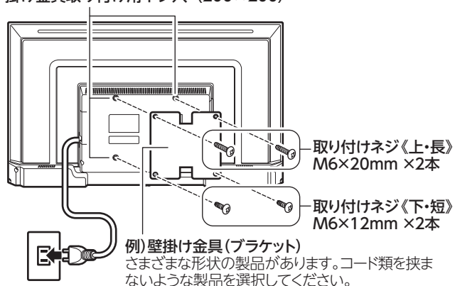
掛け金具取り付け用ネジ穴 (200×200)
