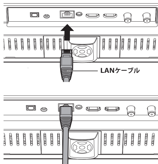
接続例
